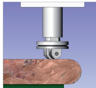
ANTISLIPPING BUSH HAMMERING (PROGRAMMABILE) BOCCIARDATURA ANTISCIVOLO (PROGRAMMABILE)
