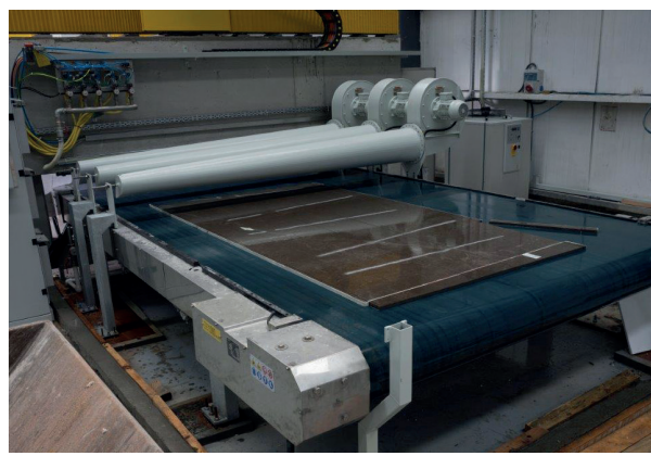
COD. 8362 Short conveyor belt for unload Nastro di scarico
